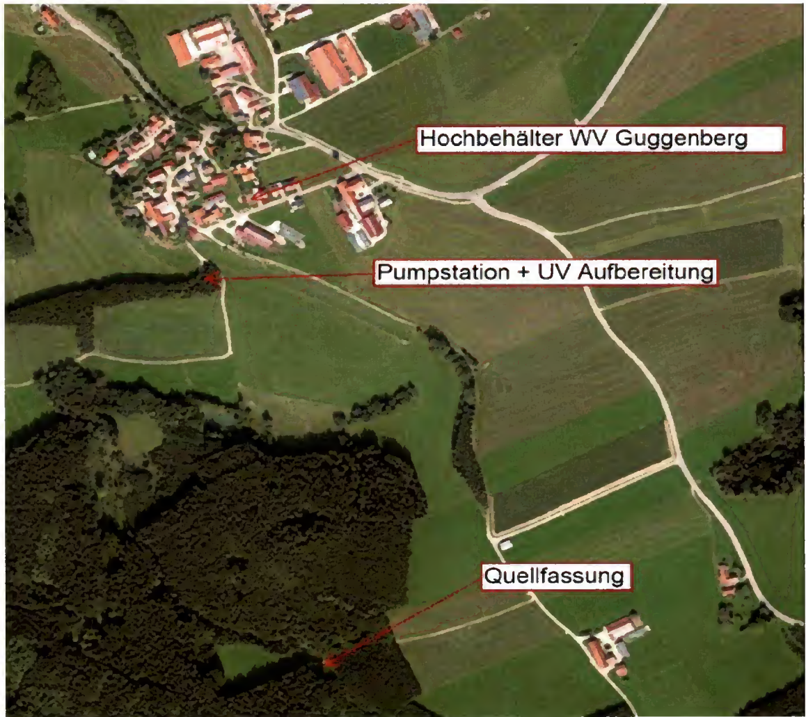
Lageplan Wasserversorgung Guggenberg M 1:8000
